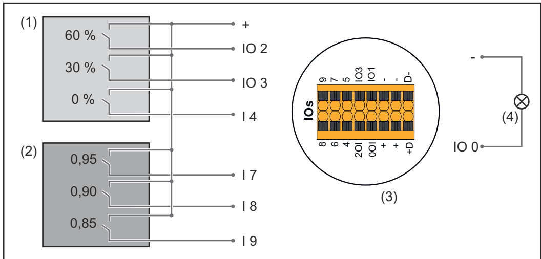
Dos receptores de telemando centralizado circular conectados a las E/S del Fronius Datamanager 2.0
