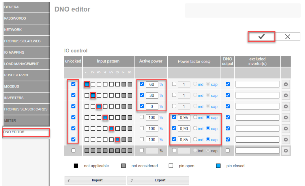
Vista general del control IO de la interfaz
