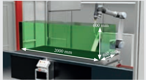
/ Bauteildimensionen: 1 Station
