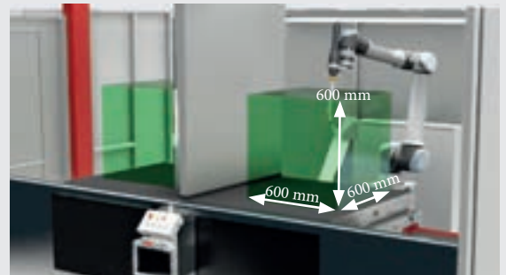
/ Bauteildimensionen: 2 Stationen
