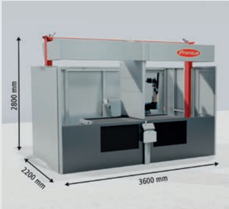
/ Bauteildimensionen: 1 Station
