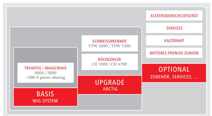
Systemüberblick ArcTig
