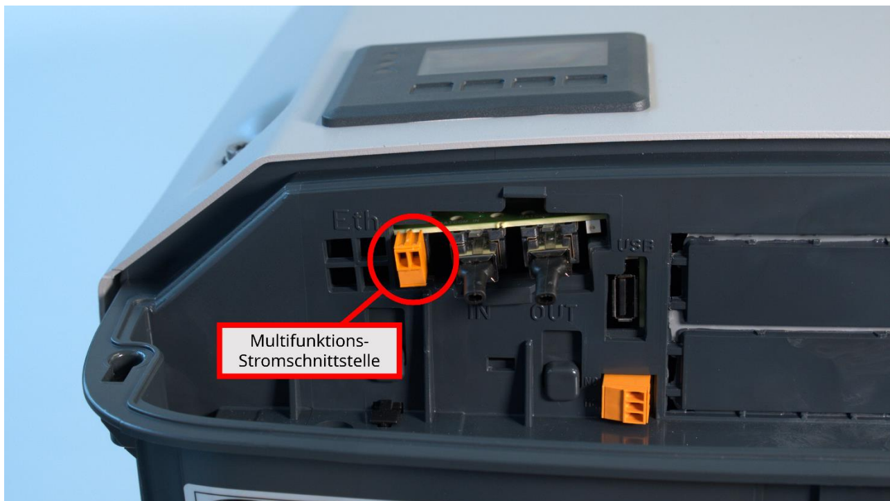
Abbildung 1: Anschlussbereich eines SnapINverter Light
