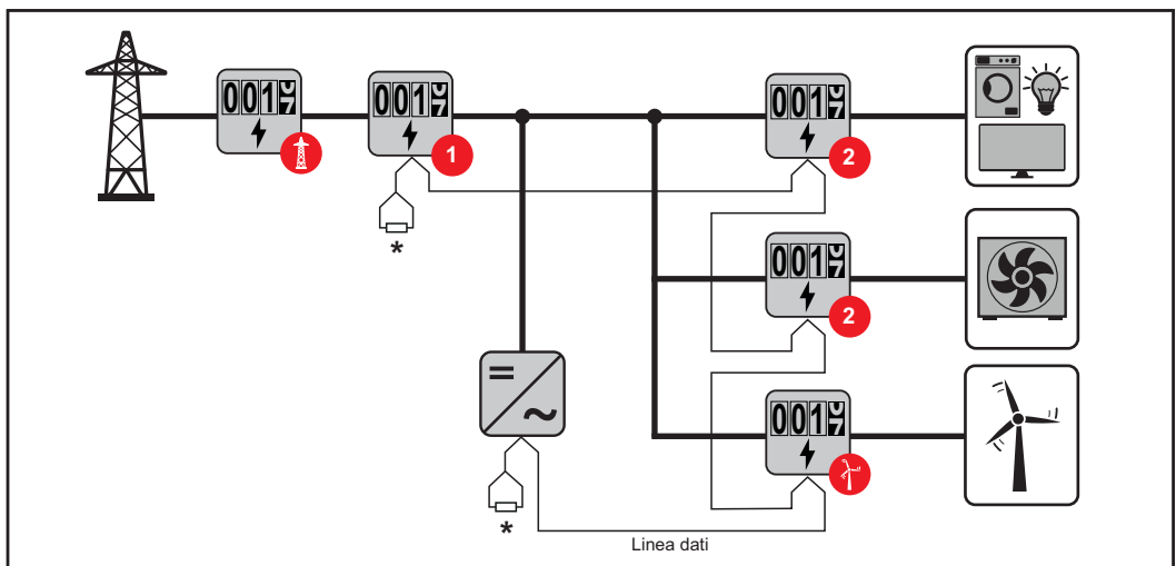
Posizione del contatore primario nel punto di alimentazione. *Resistenza terminale R 120 Ohm.
