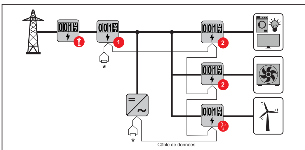
Position du compteur primaire au point d'alimentation. *Résistance terminale R 120 Ohm
