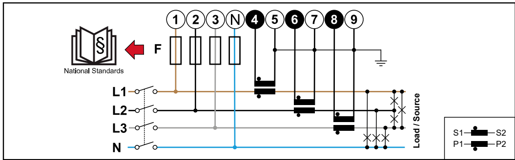
3 fazy, 4 przewody (przyłtęcze CT)
