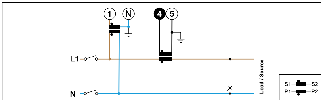
1 faza, 2 przewody (przyłącze VT/CT)
