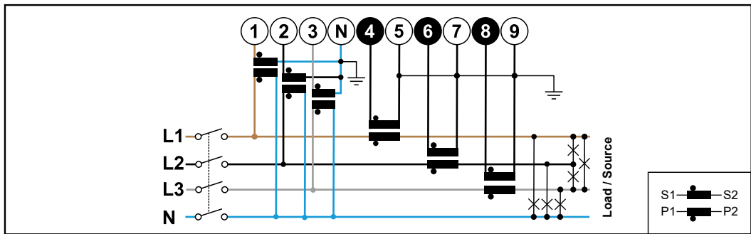
3 fazy, 4 przewody (przyłtęcze VT/CT)
