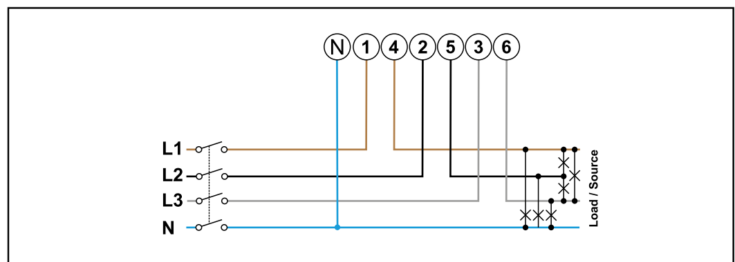
3 faze, 4 conductori
