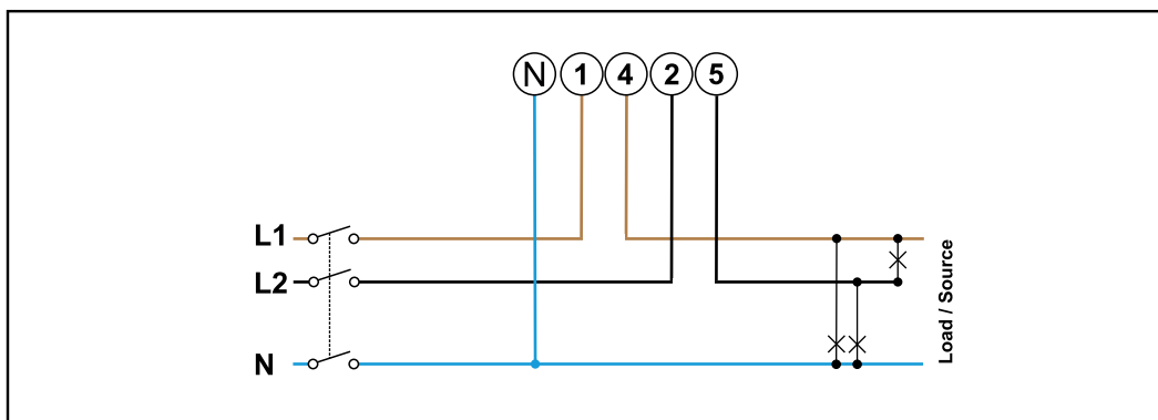
2 faze, 3 conductori
