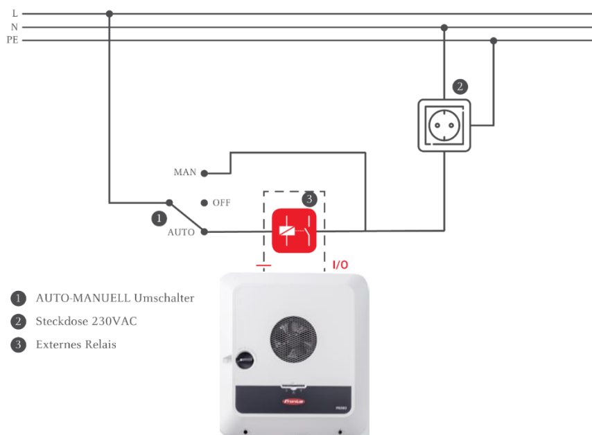
Abbildung 1 – Beispiel Schaltplan
