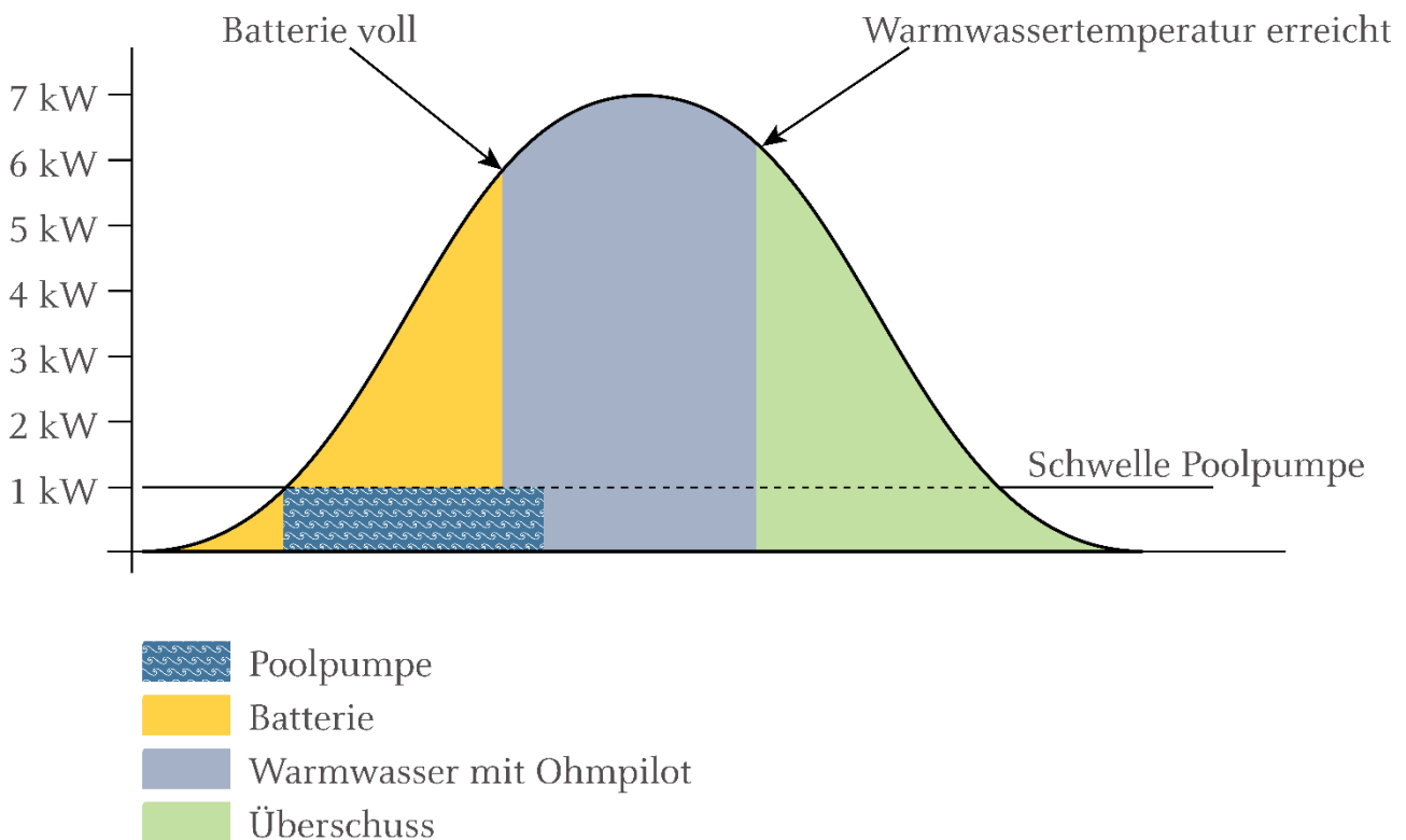
Abbildung 9 – Leistungsaufteilung
